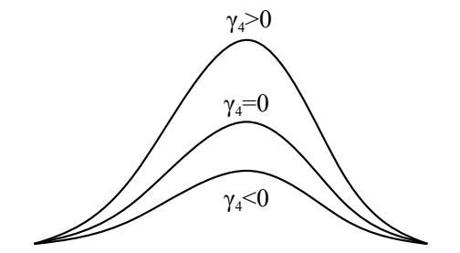
Obr. 5: Koeficient špicatosti
