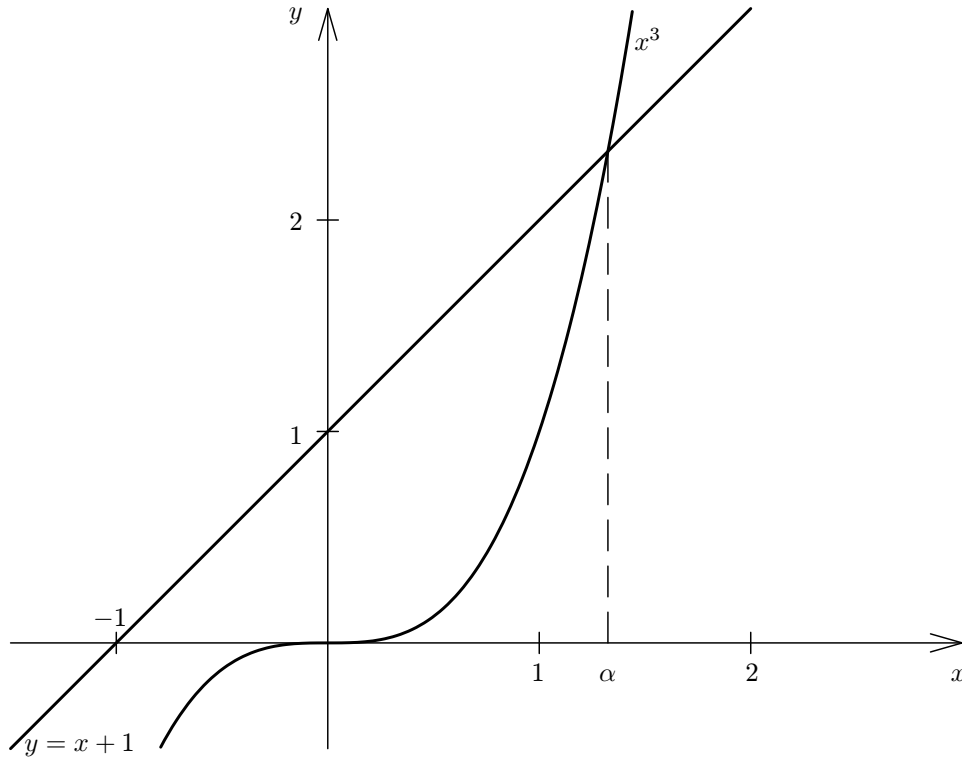
Obr. 1.1: Grafický odhad koreňov
