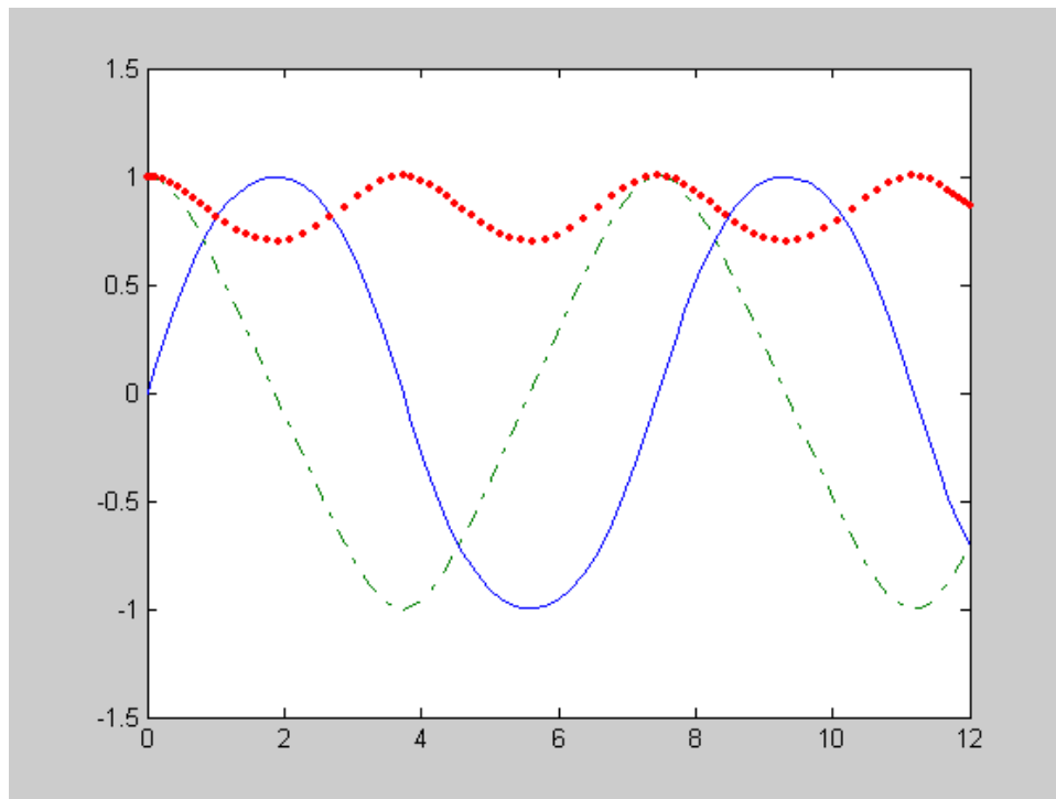
Obr. 13.2: Výsledok numerického riešenia nelineárnej sústavy diferenciálnych rovníc
