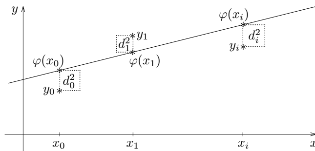
Obr. 4.2: Aproximácia pomocou lineárnej funkcie
