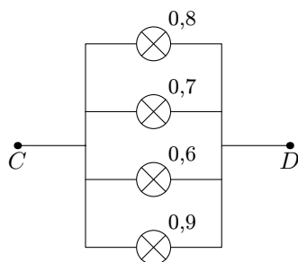
Obr. 7.2: Paralelné zapojenie
