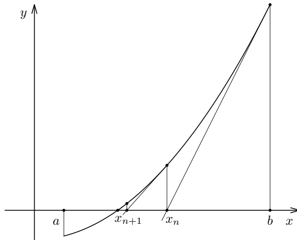
Obr. 1.2: Newtonova metóda dotyčníc
