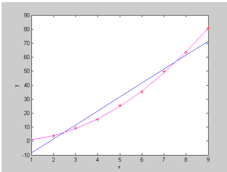
Obr. 13.1: Výsledok aproximácie v MATLABe
